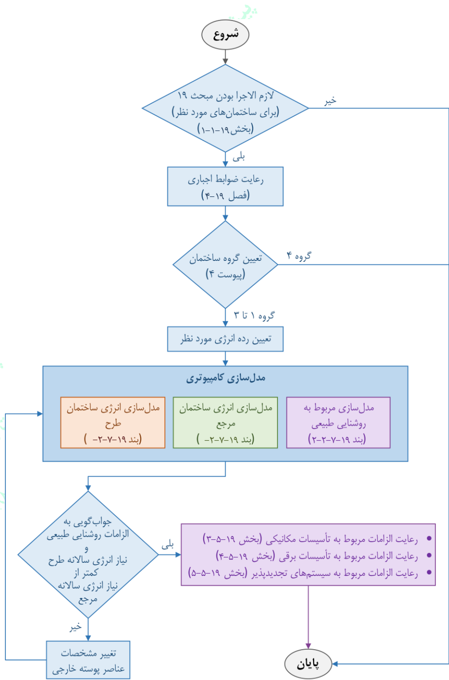
شکل ۱۹-۷-۱ نمودار گردش‌ی مراحل روش نیاز انرژی
